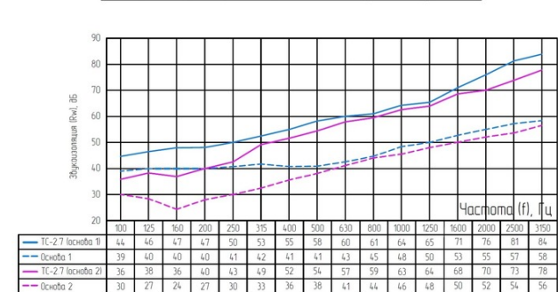
Частотные характеристики изоляции воздушного шума, R_w(f)
